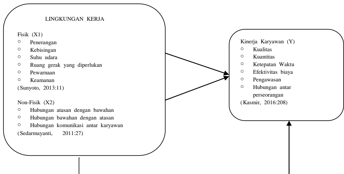
Gambar 1 Kerangka Pemikiran
